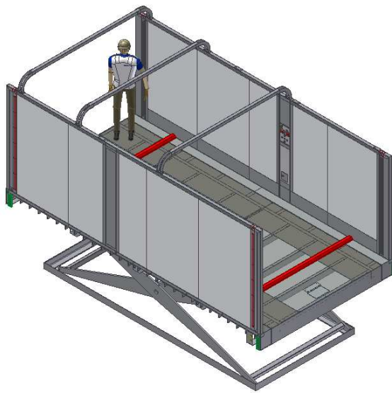
CAD 3D-ontwerp
