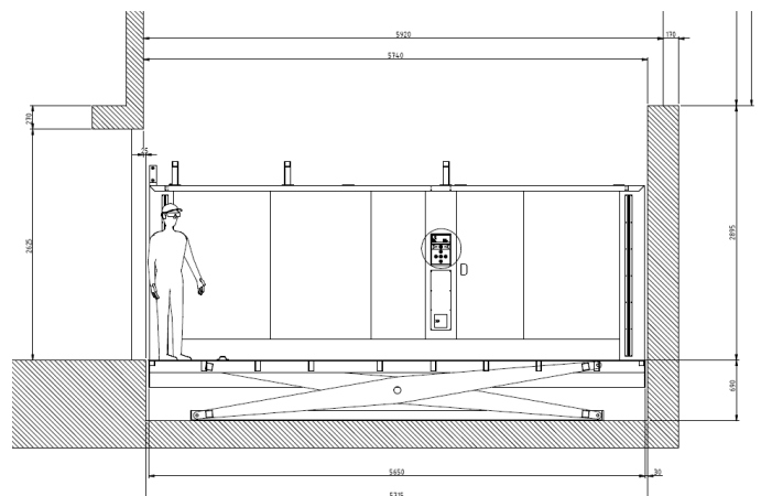
Detail: uitvoeringsplan
