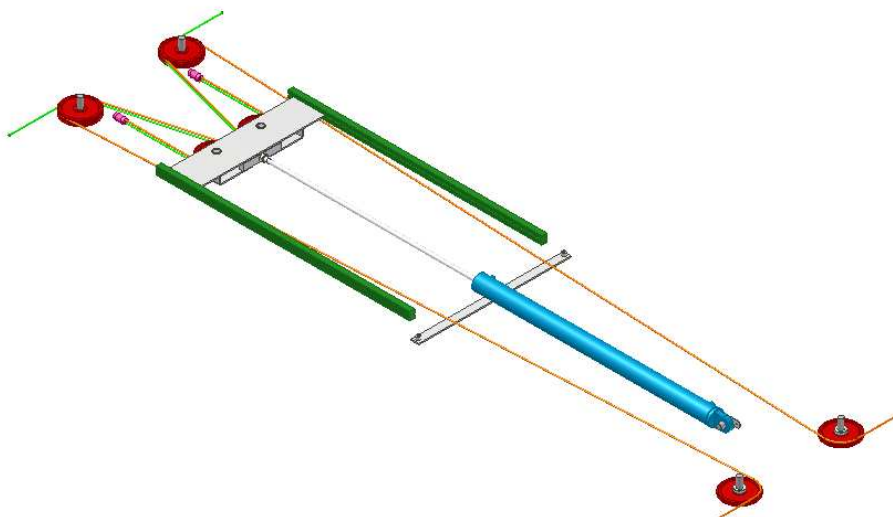
4-palensysteem: Hydraulische aandrijving met staalkabels
